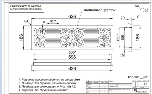
Решетка ВРК-Л «Античный цветок»
