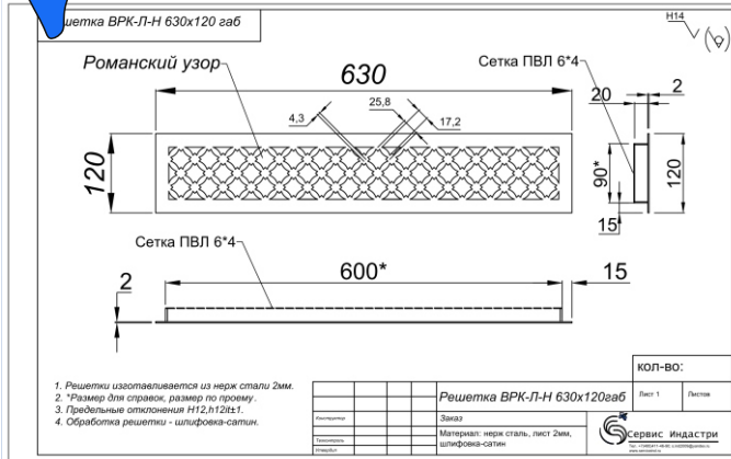
Решетка ВРК-Л-Н «Романский узор»
