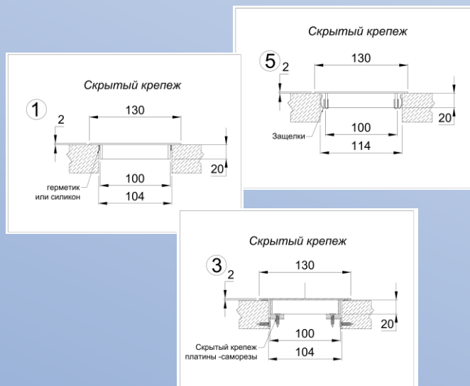
Решетка ВРК-Л-Н «Мозаика»
